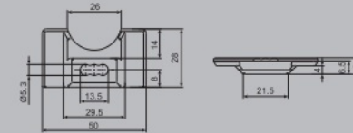
名称: 钢栓固定扣 (左右通用) 材料: 锌合金
